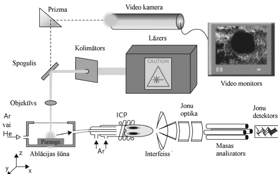
1.7. att. Lāzera ablācijas induktīvi saistītās plazmas masspektrometrija principiālā shēma (Ghent University, 2017)
