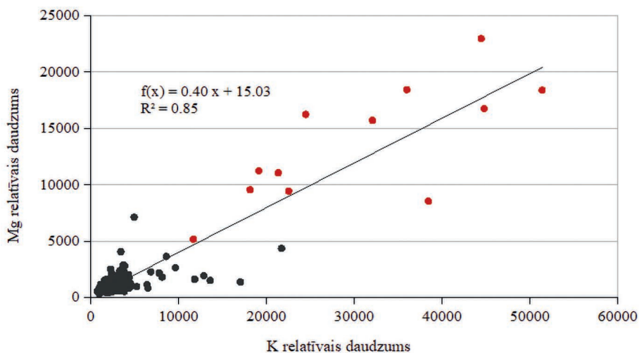
3.32. att. Sakarība starp ^{39}\text{K} un ^{26}\text{Mg} relatīvo daudzumu paraugkoka A5 gadskārtu koksne Ar pelēku krāsu apzīmētie punkti atbilst mērījumiem stubra gadskārtu koksne, ar sarkanu krāsu — vaskulārajā kambijā un iekšējā mizā
