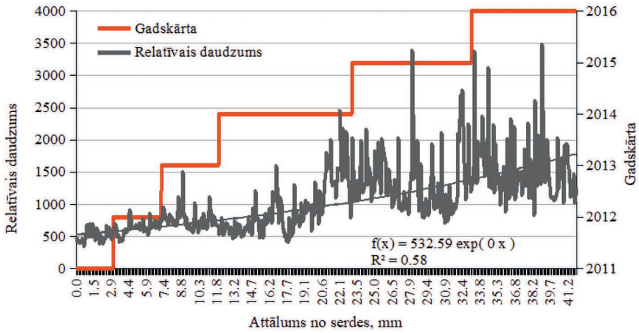
3.30. att. ^{31}\text{P} relatīvais daudzums apšu hibrīdu paraugkoka A11 gadskārtās
