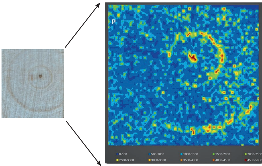
3.31. att. ^{31}\text{P} relatīvais daudzums apšu hibrīdu paraugkoka A4 pirmās trīs gadskārtās
