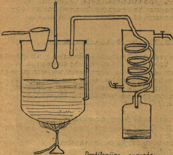
Destilazijas aparata schematisks sihmejums.
