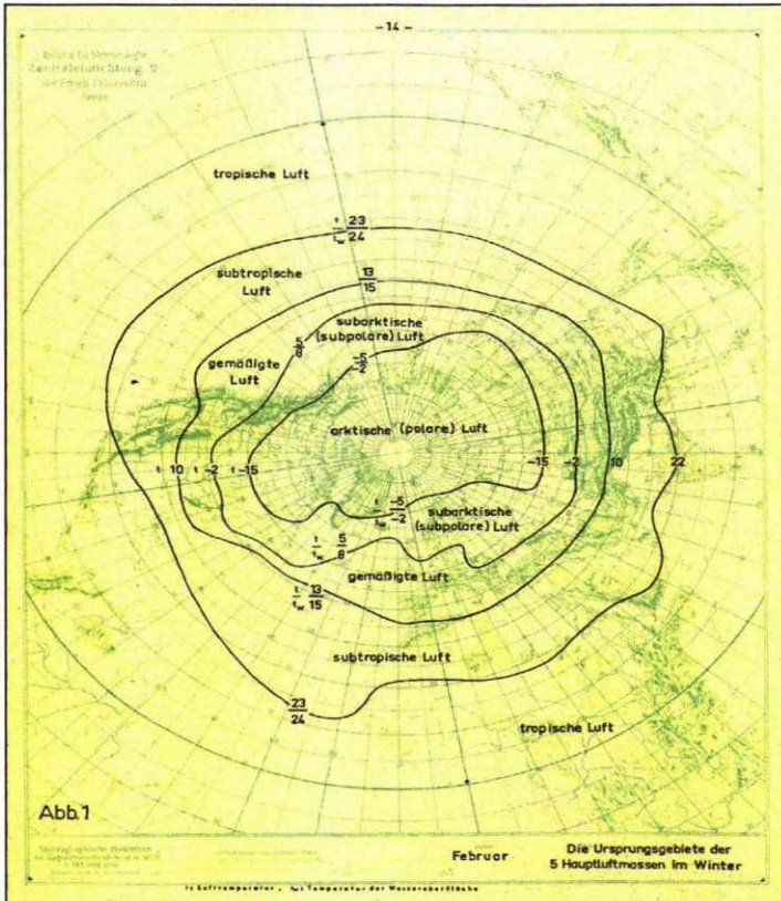
1-5. attēls. Arktisko, subpolāro, mēreno platumu/vidusplatumu (gemäßigte), subtropisko un tropisko gaisa masu veidošanās apgabali Ziemeļu puslodē ziemā (A) un vasarā (B). t/t_w – ziemas gaisa temperatūra / ūdens virsslāņa temperatūra [pēc: Geb, 1971]
