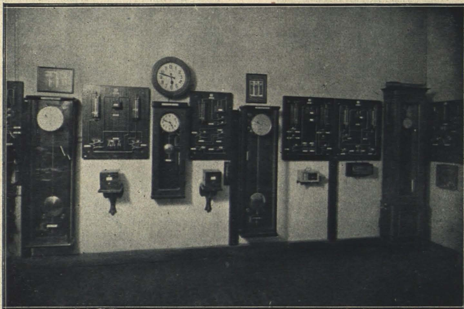
Observātorijas un laika stacijas darba pulksteņi.
