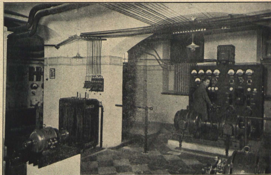
Sinchronais agregāts akumulātoru pildīšanai.
