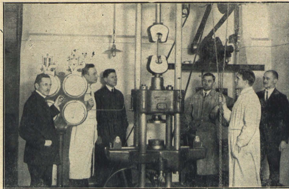
Tērauda izmēģināšana uz stiepi.
