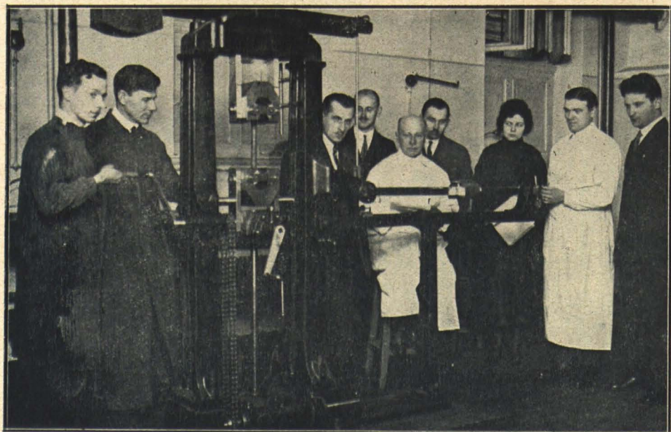
Dzelzs izmēģināšana (Losenhausen'a 5000 kg rauj. maš.).
