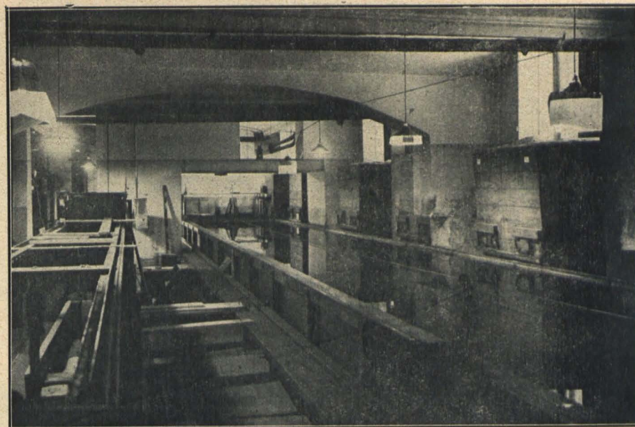
Ūdensbūvju laborātorijas ūdens straumes sile.
