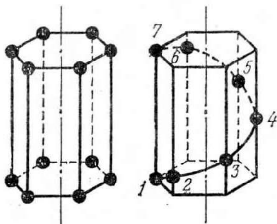
Рис. 15 Действие простой оси симметрии 6-го порядка и одной из винтовых осей того же порядка
