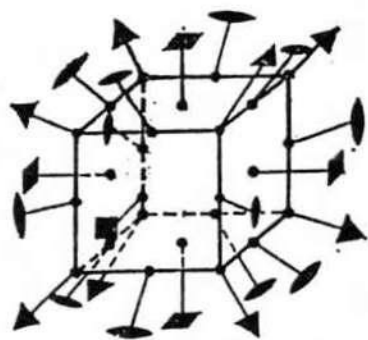
Рис. 4. Все оси симметрии куба
