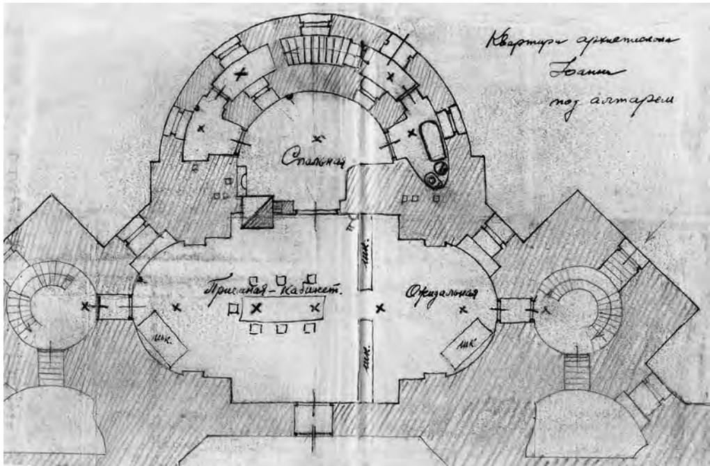
План квартиры архиепископа Иоанна под алтарем Кафедрального собора. В. Шервинский
