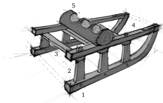
3. zīm. Baļķu ragaviņas. 1 – sliece, 2 – mietne, 3 – balziens, 4 – uzkala, 5 – kūlenis. Zīm. J. Z. Jātnieks, 2025
