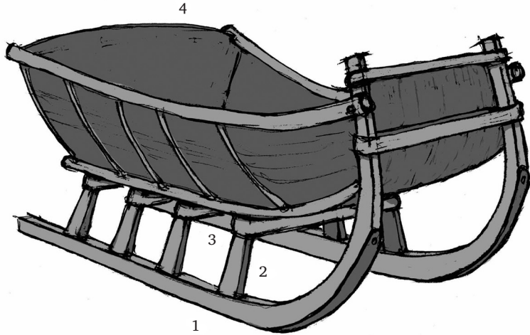
2. zīm. Ragavas ar laivveida kulbu. 1 – sliece, 2 – mietne, 3 – balziens, 4 – kriju kulba. Zīm. J. Z. Jātnieks, 2025
