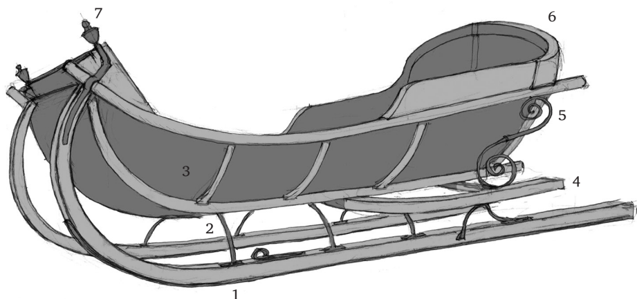
4. zīm. 20. gs. 20.–30. gados profesionāla amatnieka izgatavotas kamanas ar vienlaidus kulbu. 1 – liektas slieces, 2 – apaļmetāla mietnes, 3 – kulba, 4 – spārniņi, 5 – dekoratīvi izliekts kulbas un spārniņu stiprinājums, 6 – noapaļotas formas kulbas atzveltne, 7 – sniegtveris ar abās pusēs dekoratīvi stiprinātu misiņa dekoru. Zīm. J. Z. Jātnieks, 2025
