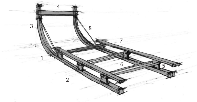
1. zīm. Ragavu pamatkonstrukcija. 1 – liektas slieces, 2 – slieču ceļa daļas metāla apkalums, 3 – apgalvenis, 4 – šķērsis, 5 – mietne, 6 – balziens, 7 – uzkala, 8 – atstope. Zīm. J. Z. Jātnieks, 2025
