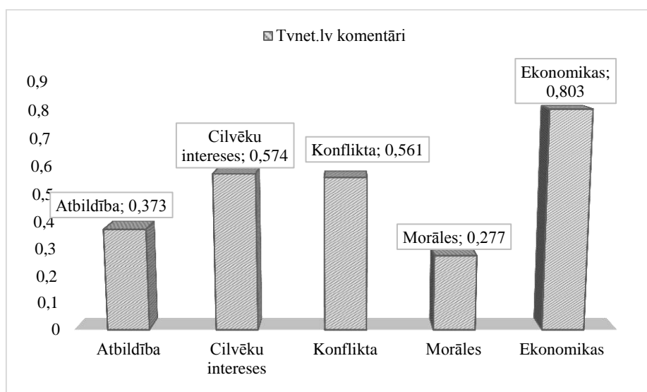
3.15. att. Analīzē izmantojamo tvnet.lv komentāru Kronbaha alfa
